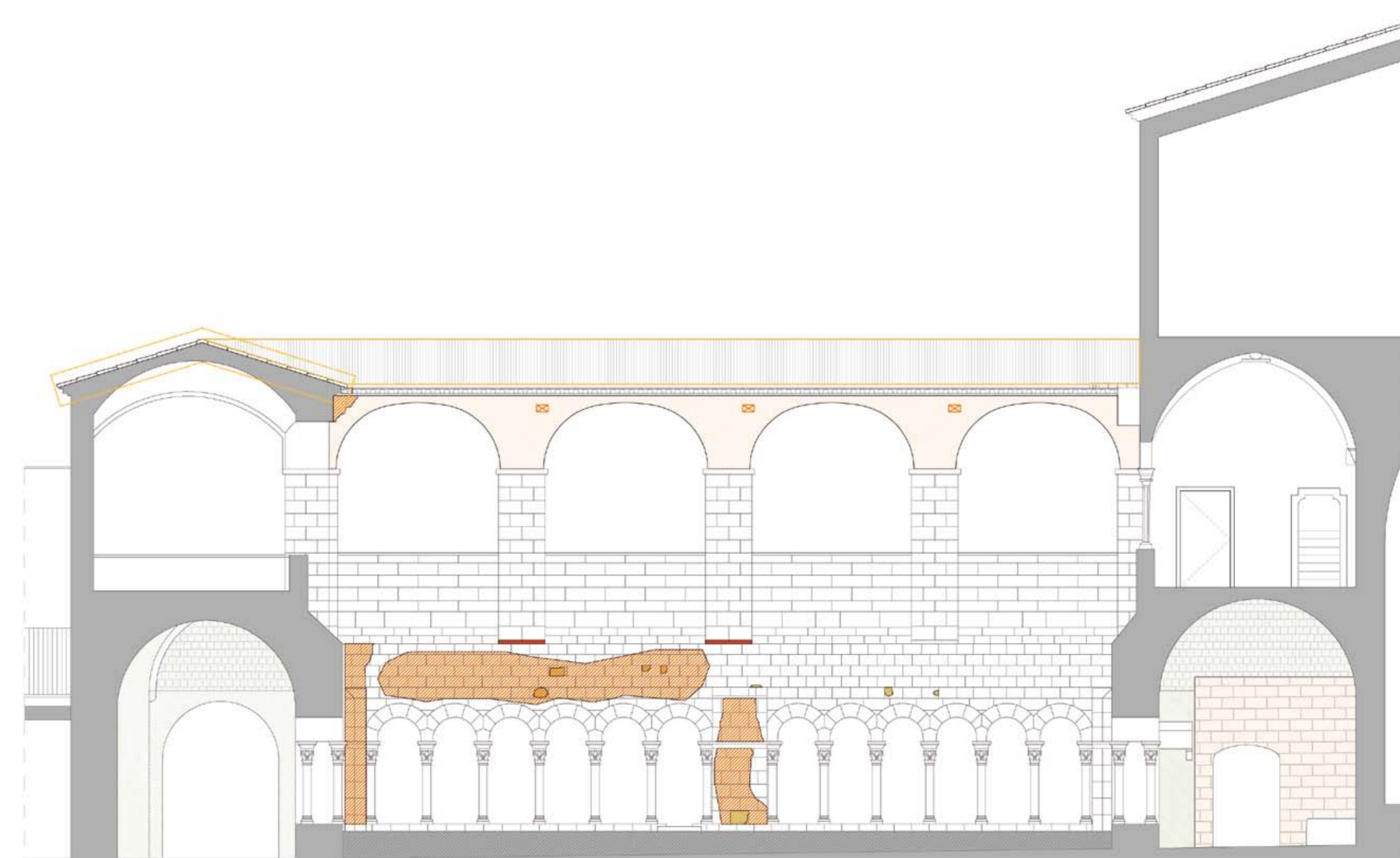
ALÇAT MUR INTERIOR OEST
