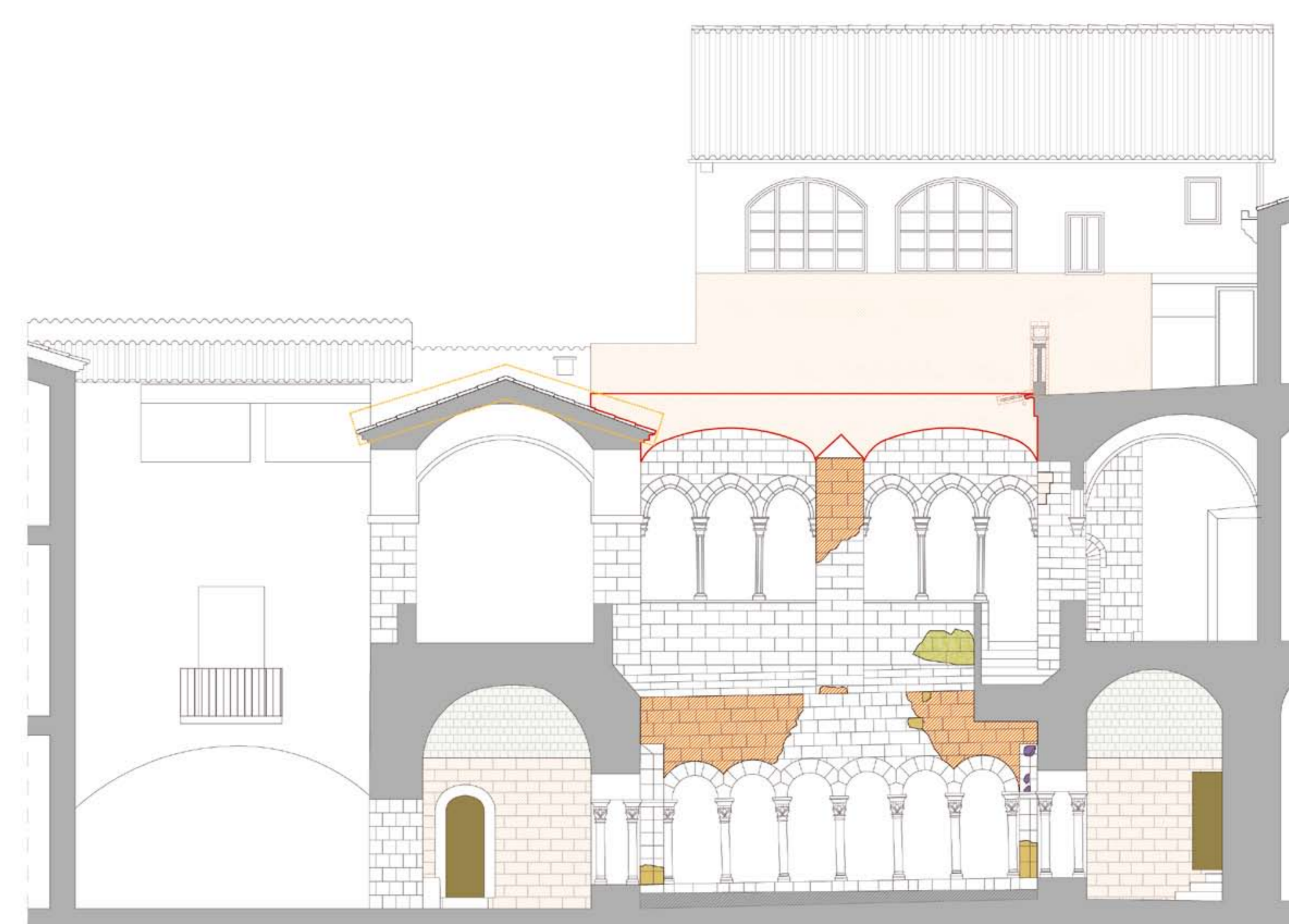
ALÇAT MUR INTERIOR NORD
