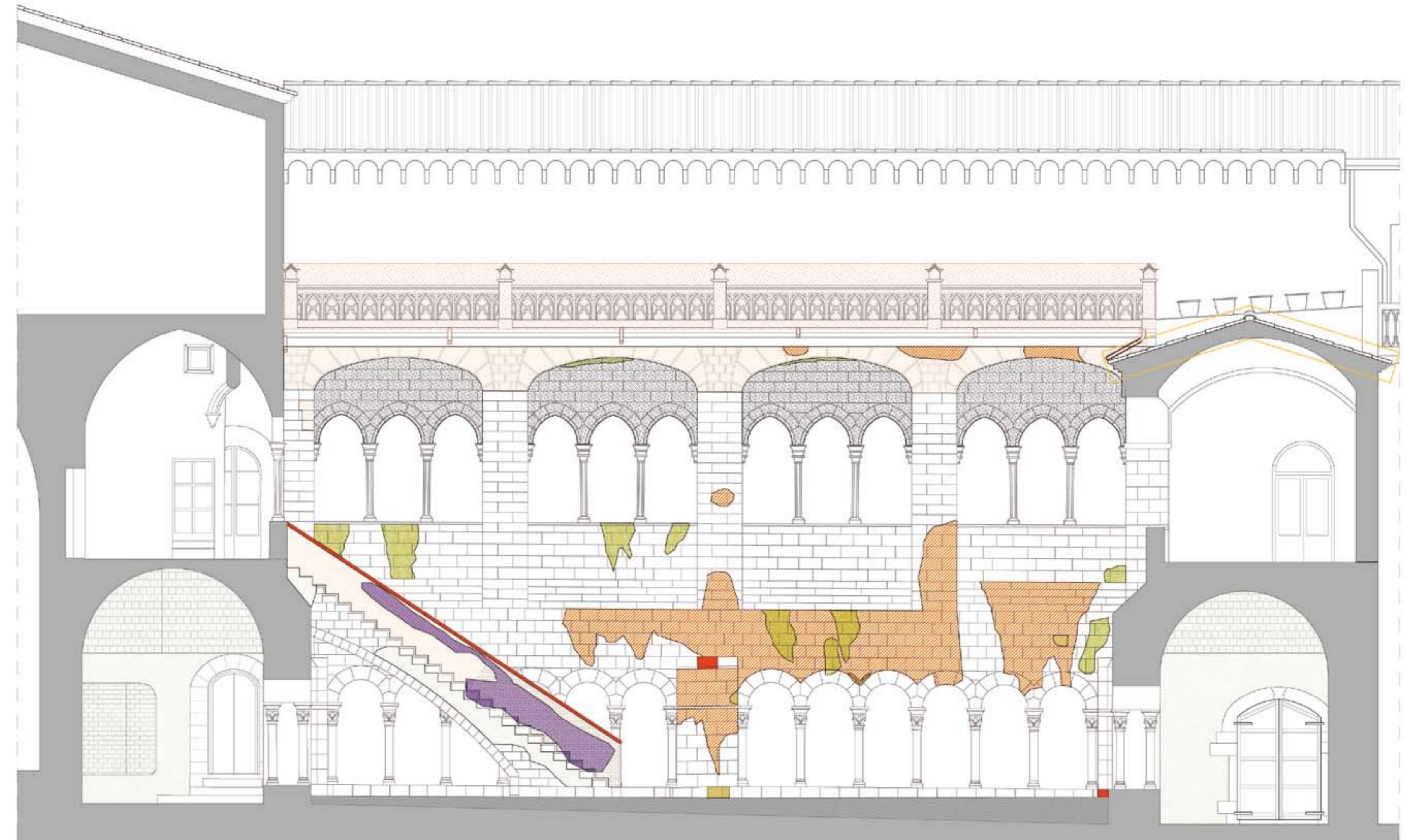
ALÇAT MUR INTERIOR EST 2
