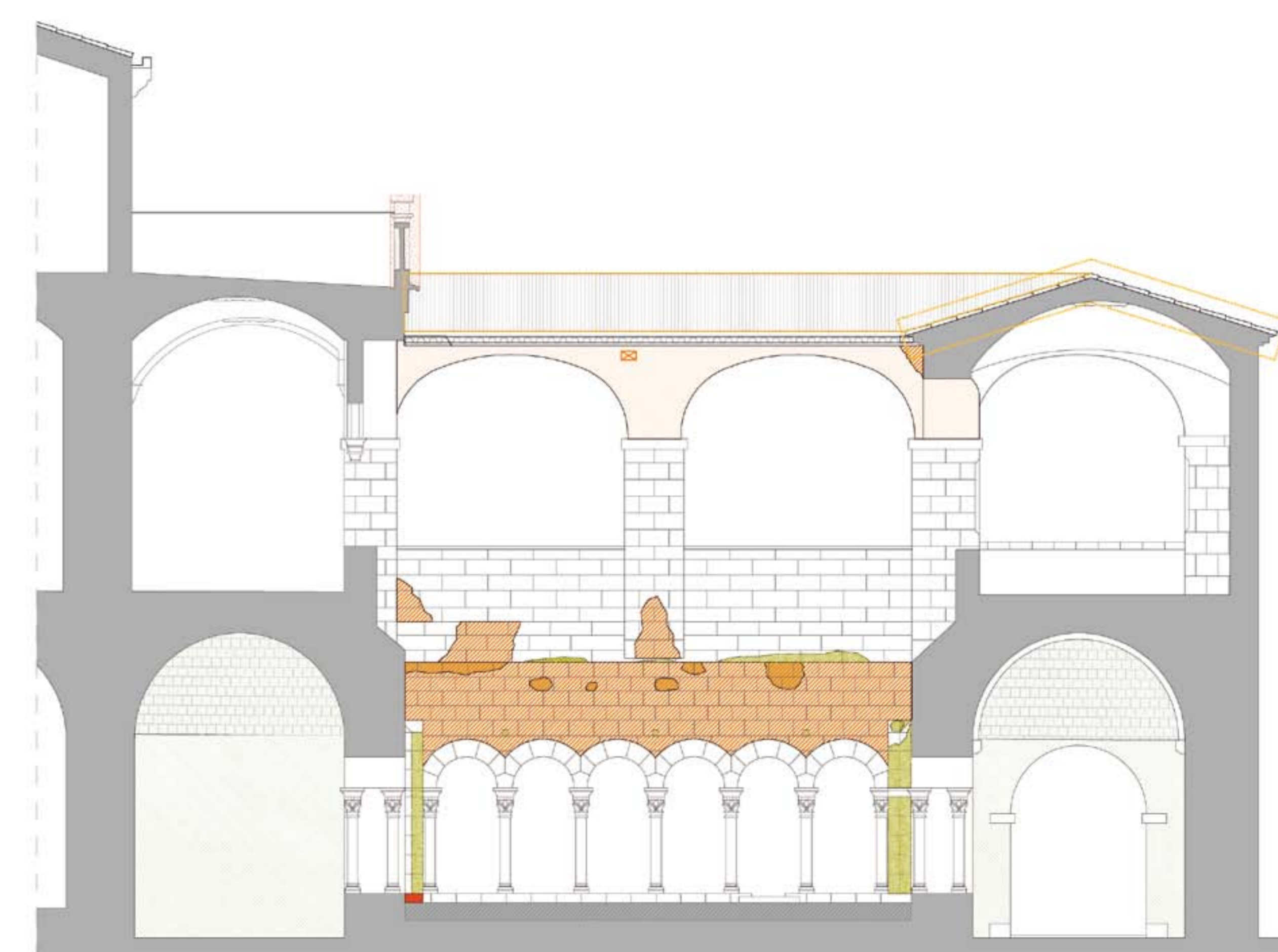
ALÇAT MUR INTERIOR SUD
